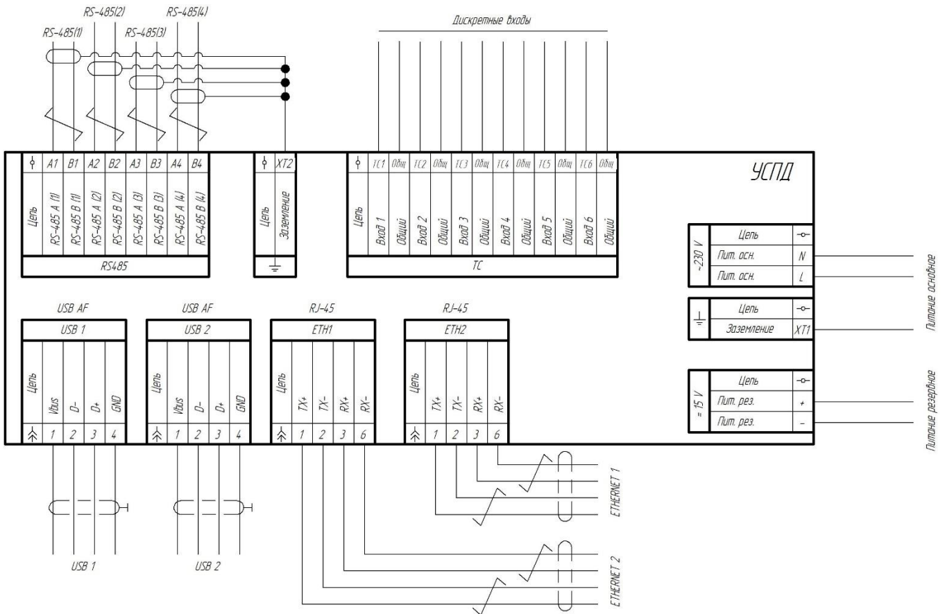
Рисунок Б.2 - Схема подключения УСПД
